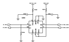
UART Level Shifter
