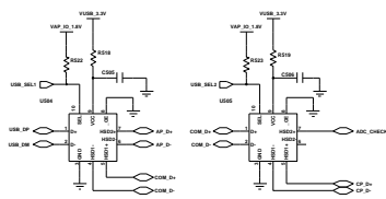
USB SWITCH IC
